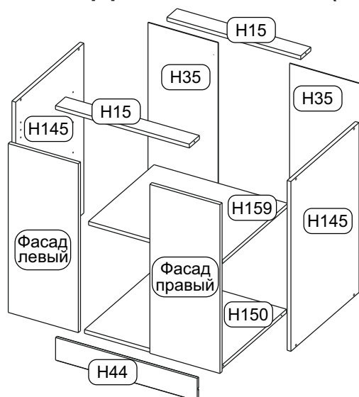
Шкаф рабочий L800 В500 (2 дв.)
